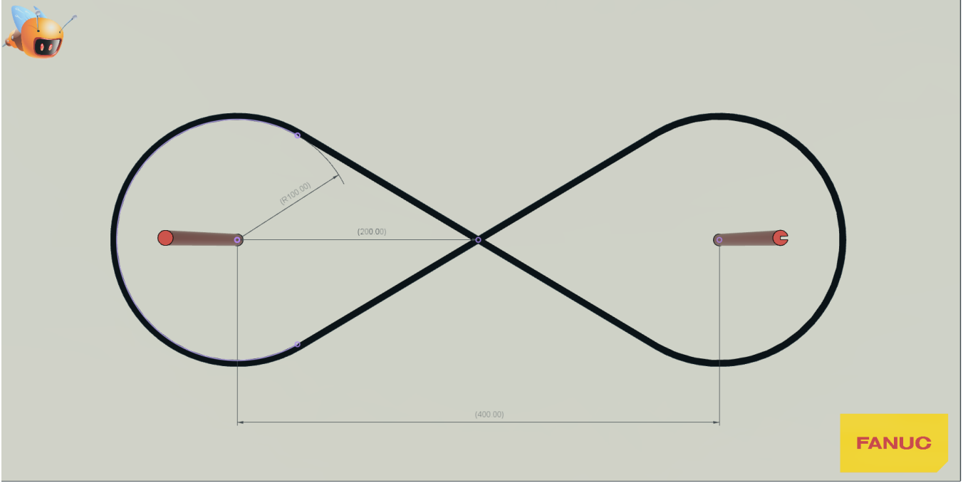
Şekil 1 – Yarış pistinin üstten görünümü ve boyutları
